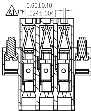
SEC A-A
